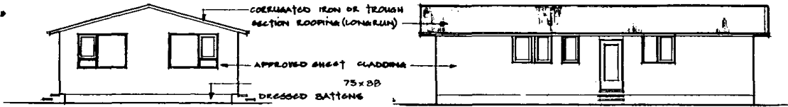
ELEVATION 1
