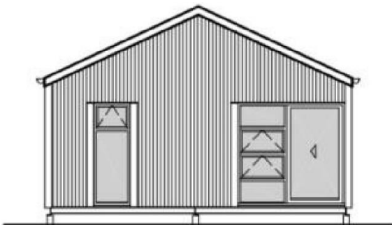
ELEVATION B
